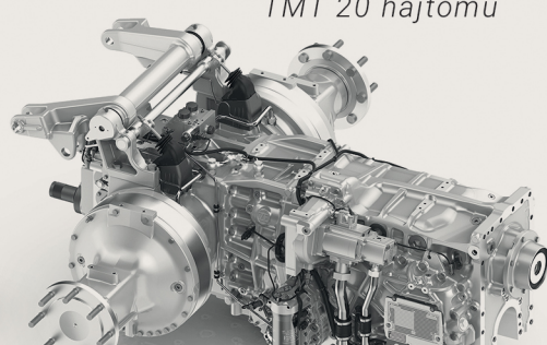
ZF TERRAMATIC TMT 20 hajtómű
