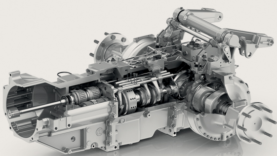
ZF TERRAMATIC hajtómű
