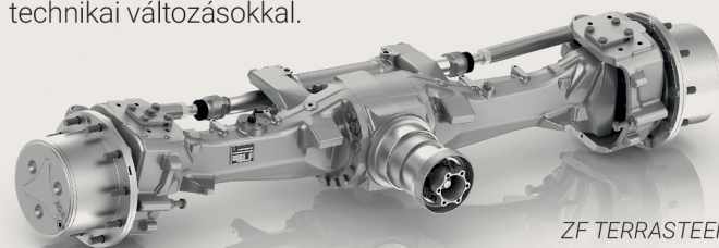
kormányzott hajtott tengely
