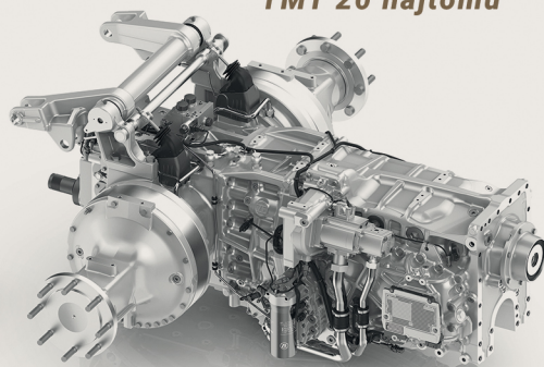
ZF TERRAMATIC TMT 20 hajtómű
