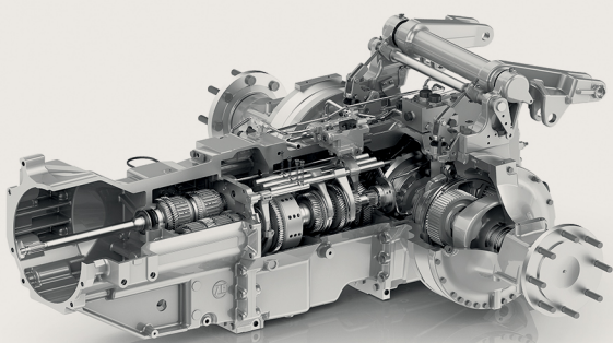
ZF TERRAMATIC hajtómű
